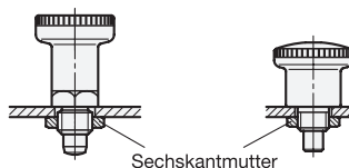
Rastbolzen GN 607 / GN 607.1
