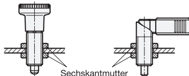
Rastbolzen GN 613
